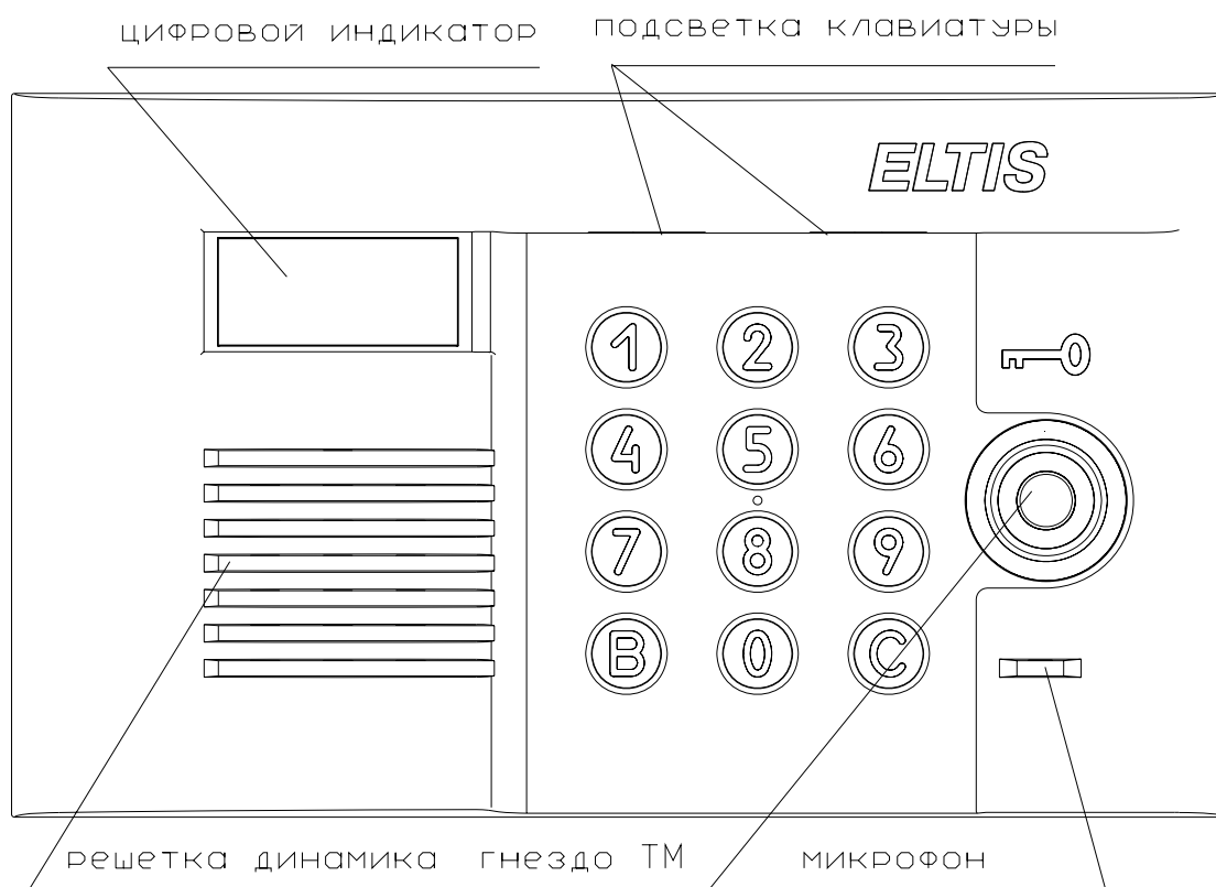
Рис.1 Внешний вид со стороны лицевой панели блока вызова DP303-TD16.
